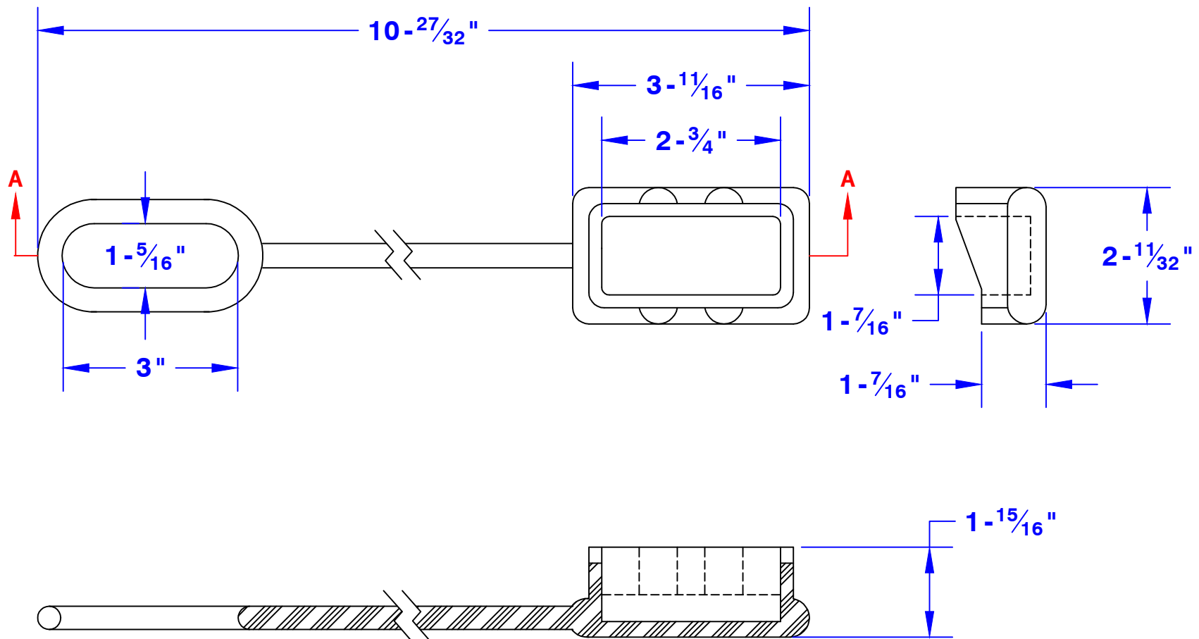
Section A-A
